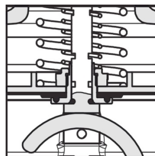
Рисунок 3: версия С сбросным клапаном
