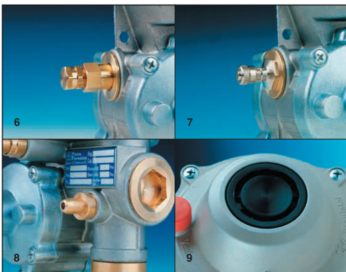
6. ШТУЦЕР ОТБОРА ИМПУЛЬСА ТИПА PETERSON INLET TEST POINT - TYPE PETERSON
