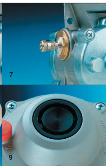
7. ШТУЦЕР ОТБОРА ИМПУЛЬСА ТИПА Ø7,7X0,794 INLET TEST POINT - TYPE Ø 7,7X0,794
