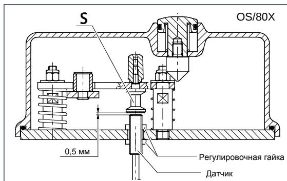
Установка пилота
