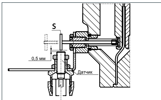
Установка регулятора/монитора
